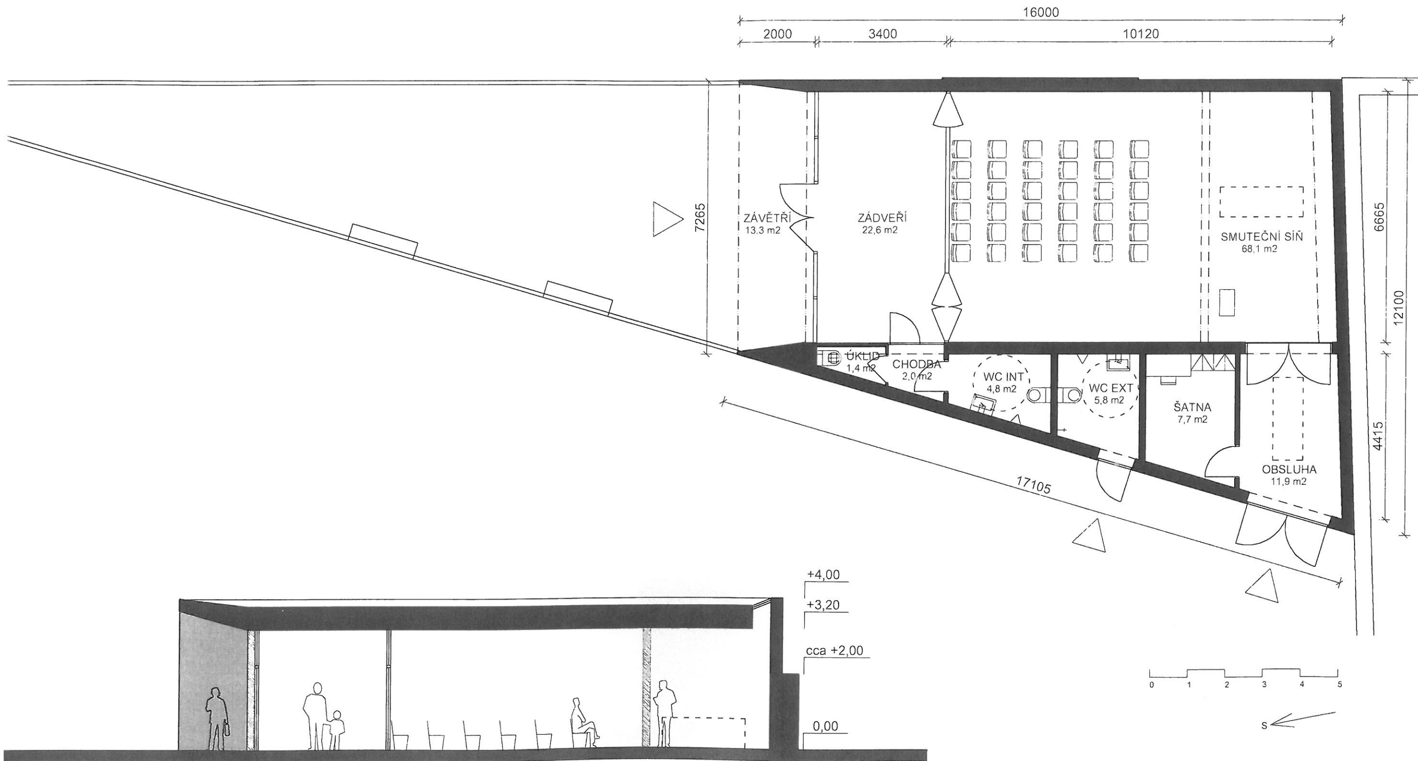
ŘEZ PODÉLNÝ
